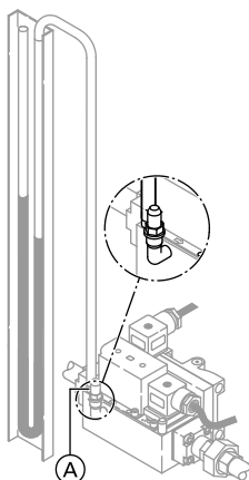
Комбинированная газовая арматура, производитель Kromschröder
