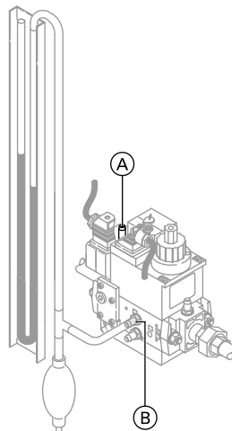
Комбинированная газовая арматура, производитель Dungs
